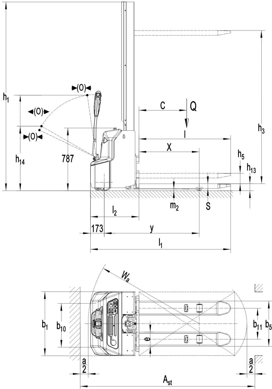
Fig. 2 : Données techniques
